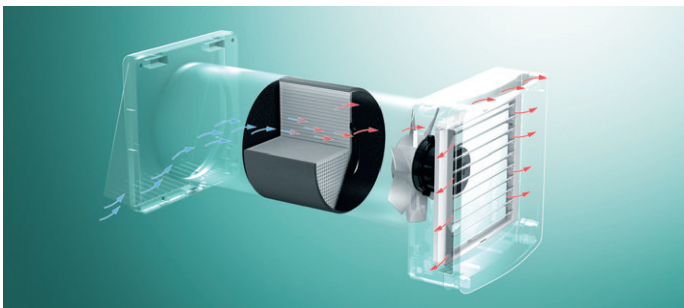
Odzysk ciepła w ceramicznym wymienniku
