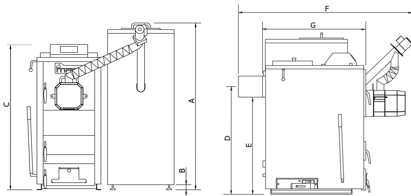
Rysunek 2. Podstawowe wymiary kotła MPM Wood Pell
